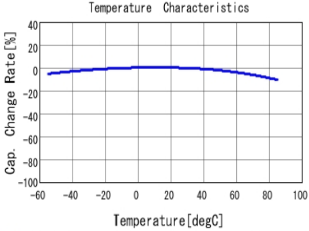
■ GRM155R61A224KE19 C-Temp. capchange, DCO. 0V, ACO. 5V rm
