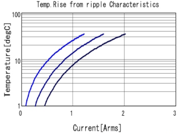
GRM155R61A224KE19 Temp. rise ■ 100kHz ■ 500kHz ■ 1MHz
