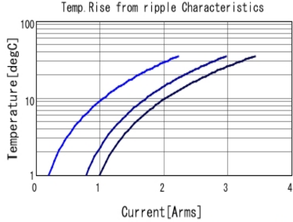
GRM155R61A105KE15 Temp. rise ■ 100kHz ■ 500kHz ■ 1MHz
