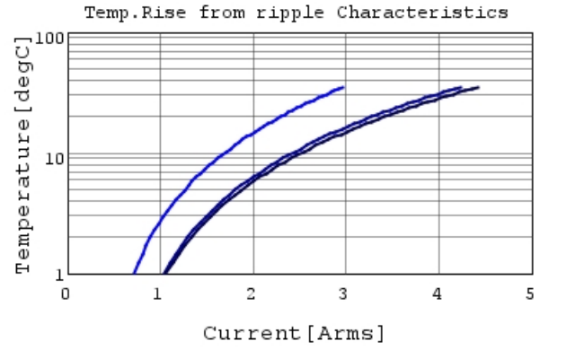
GRM155R60J475ME87 Temp.rise — 100kHz —
