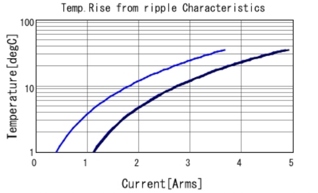
GRM155R60J475ME47 Temp. rise — 100kHz — 500
