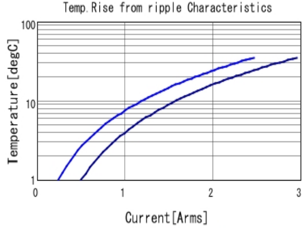
GRM155R60J105KE19 Temp. rise ■ 500kHz ■ 1MHz
