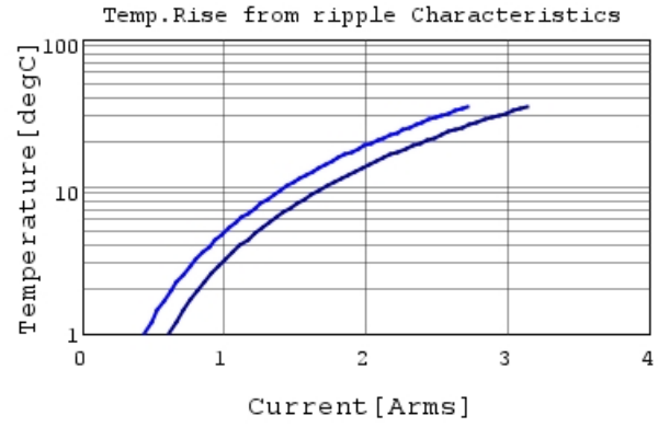
GRM155C81E105KE11 Temp.rise 500kHz
