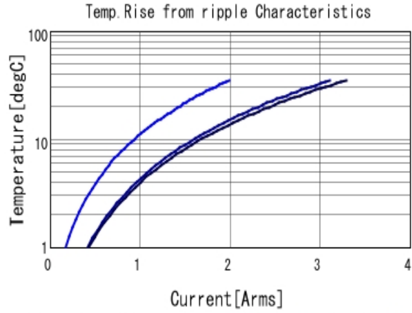
GRM155C81A225KE44 Temp. rise ■ 100kHz ■ 500kHz ■ 1MHz
