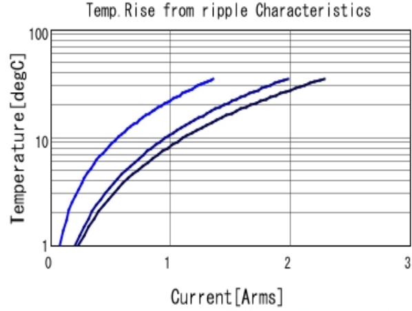
GRM155C81A105KA12 Temp. rise ■ 100kHz ■ 500kHz ■ 1MHz
