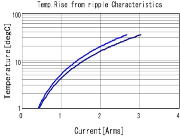
GRM155C71A105KE11 Temp. rise ■ 500kHz ■ 1MHz
