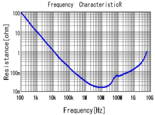
■ GRM155B31H104KE14 R DCOV, 20degC
