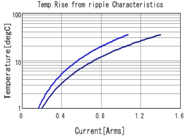
GRM155B31H104KE14 Temp. rise ■ 500kHz ■ 1MHz
