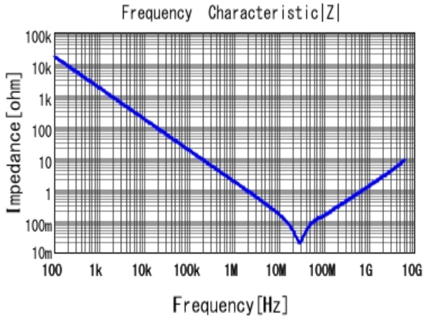
■ GRM155B31H104KE14 |Z| DCOV, 20degC
