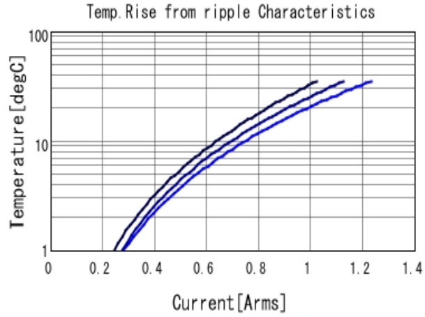
GRM1555C2A470JA01 Temp. rise ■ 500MHz ■ 700MHz ■ 1GHz
