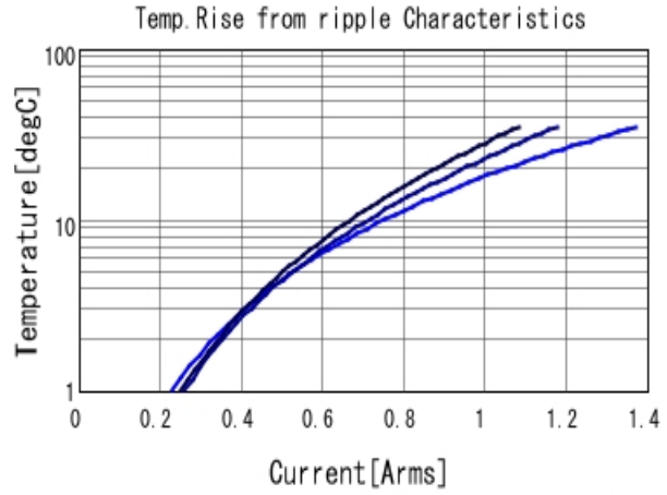
GRM1555C2A101JA01 Temp. rise ■ 200MHz ■ 500MHz ■ 700M
