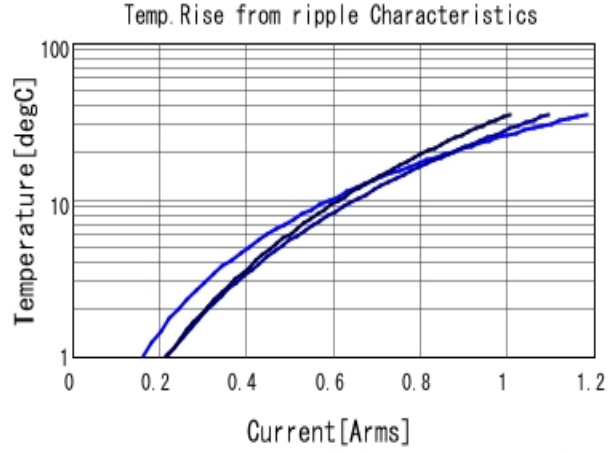
GRM1555C1H820GA01 Temp. rise ■ 200MHz ■ 500MHz ■ 700M
