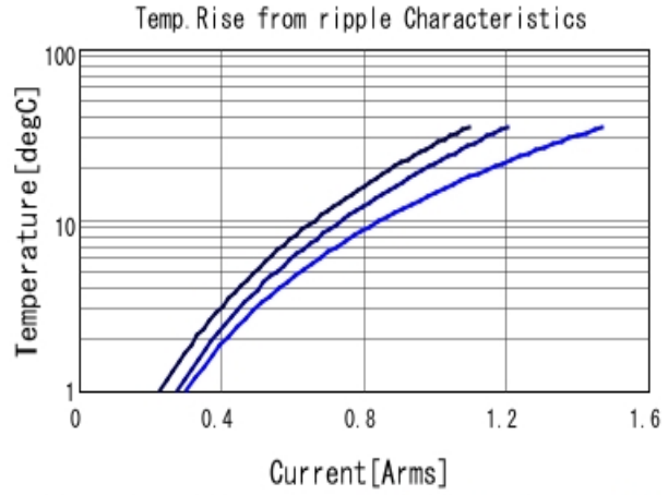
GRM1555C1H560JA01 Temp. rise ■ 200MHz ■ 500MHz ■ 700M
