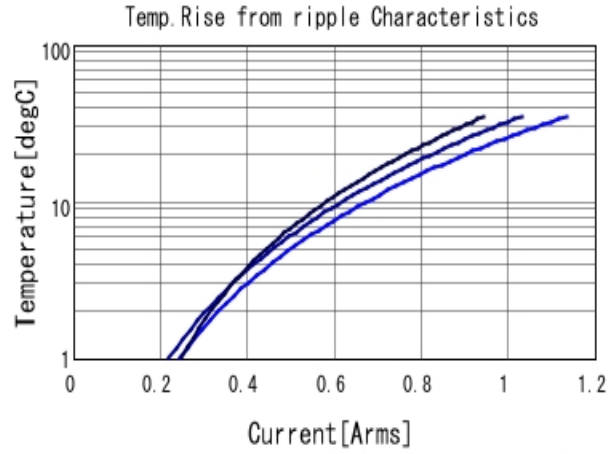
GRM1555C1H430JA01 Temp. rise ■ 500MHz ■ 700MHz ■ 1GHz
