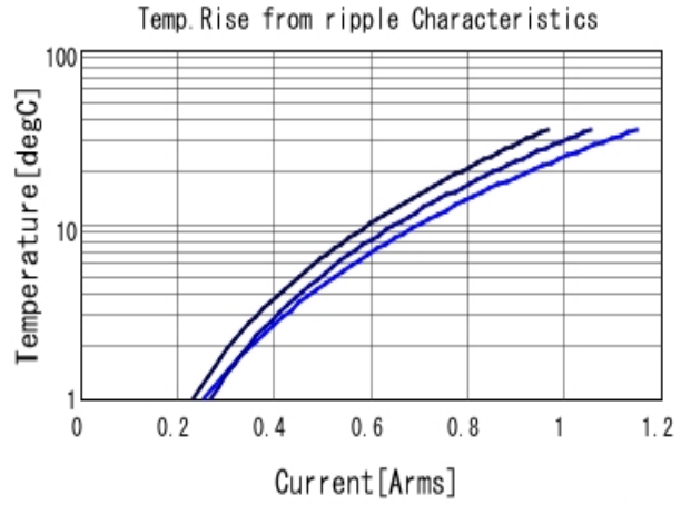
GRM1555C1H390JA01 Temp. rise ■ 500MHz ■ 700MHz ■ 1GHz
