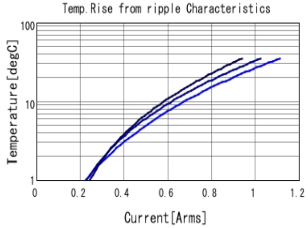
GRM1555C1H270GA01 Temp. rise ■ 500MHz ■ 700MHz ■ 1GHz
