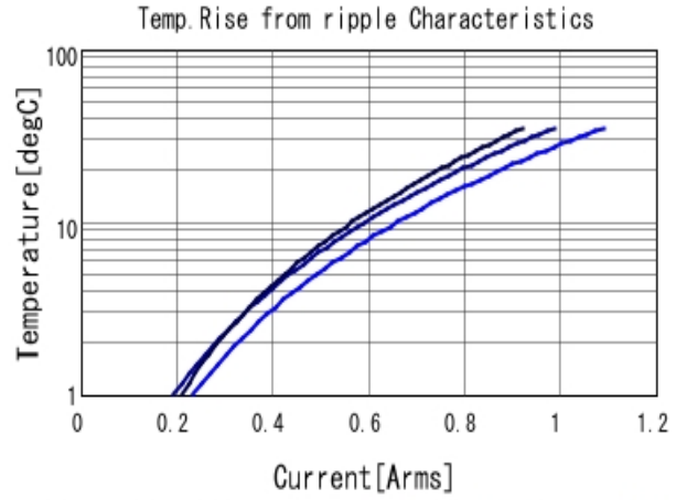
GRM1555C1H220JA01 Temp. rise ■ 500MHz ■ 700MHz ■ 1GHz
