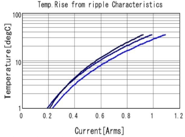
GRM1555C1H220GA01 Temp. rise ■ 500MHz ■ 700MHz ■ 1GHz
