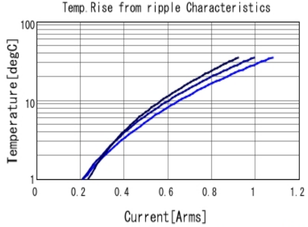
GRM1555C1H200JA01 Temp. rise ■ 500MHz ■ 700MHz ■ 1GHz
