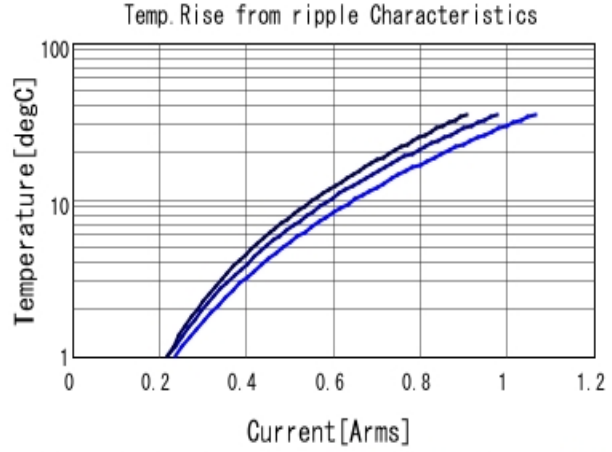
GRM1555C1H180GA01 Temp. rise ■ 500MHz ■ 700MHz ■ 1GHz
