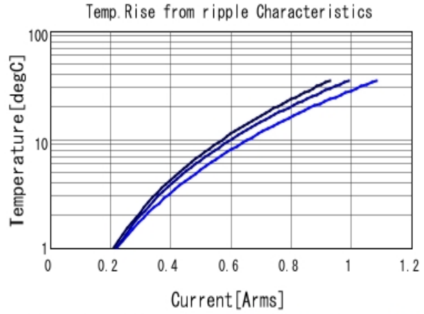
GRM1555C1H160JA01 Temp. rise ■ 500MHz ■ 700MHz ■ 1GHz
