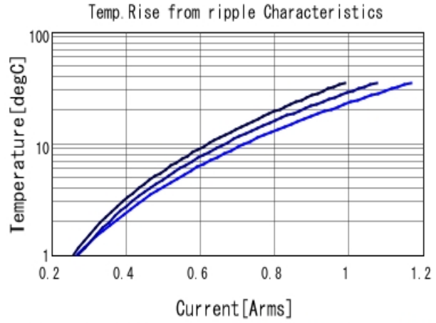
GRM1555C1H150JA01 Temp. rise ■ 500MHz ■ 700MHz ■ 1GHz
