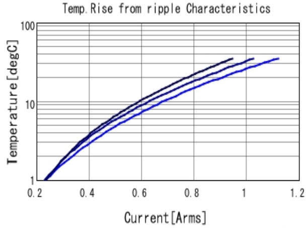
GRM1555C1H130JA01 Temp. rise ■ 500MHz ■ 700MHz ■ 1GHz
