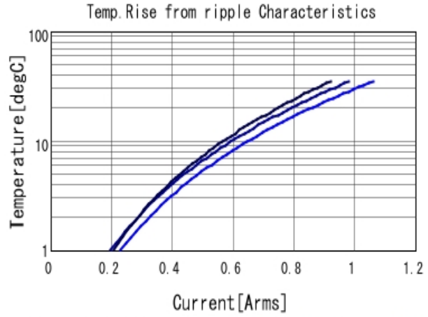
GRM1555C1H120JA01 Temp. rise ■ 500MHz ■ 700MHz ■ 1GHz
