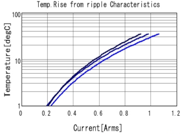
GRM1555C1H120GA01 Temp. rise ■ 500MHz ■ 700MHz ■ 1GHz
