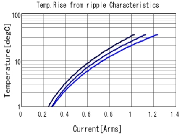
GRM1555C1E470JA01 Temp. rise ■ 500MHz ■ 700MHz ■ 1GHz
