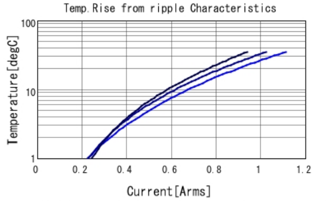
GRM1555C1E270JA01 Temp. rise — 500MHz — 700I
