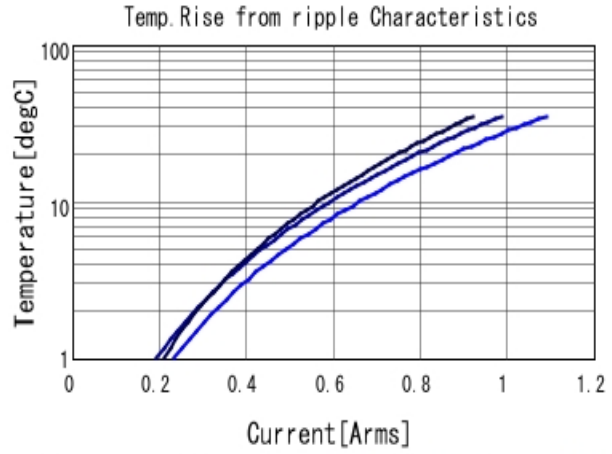
GRM1555C1E220JA01 Temp. rise ■ 500MHz ■ 700MHz ■ 1GHz
