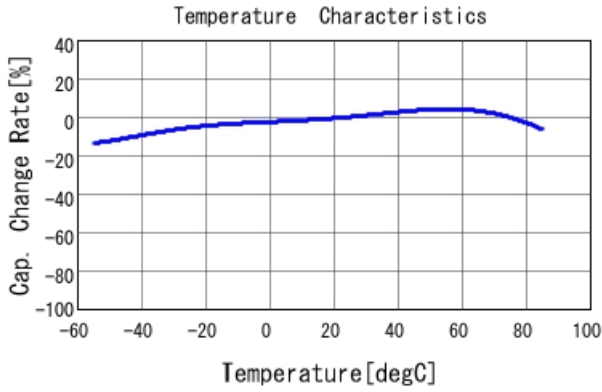
■ GRM153R61A105ME95 C-Temp. capchange, DCO. 0V, ACO. 2Vrm
