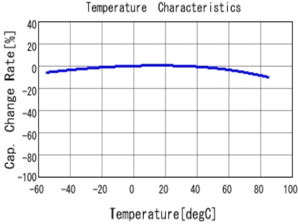
■ GRM152R61A104KE19 C-Temp. capchange, DCO. 0V, ACO. 5V rm
