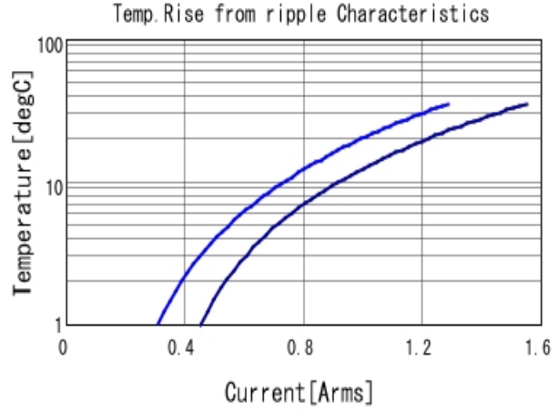
GRM152R61A104KE19 Temp. rise ■ 500kHz ■ 1MHz
