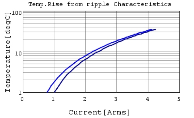
GRM035R60J475ME15 Temp.rise — 500kHz
