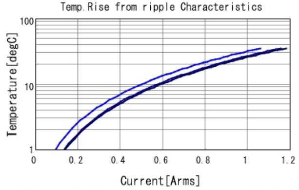
GRM033R6YA104KE14 Temp. rise ■ 400kHz ■ 800kHz ■ 1MHz
