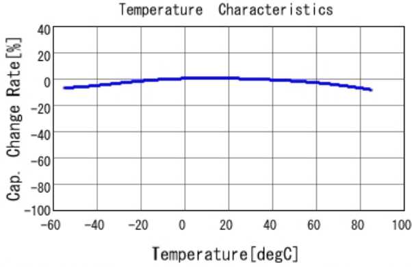
■ GRM033R6YA104KE14 C-Temp. capchange, DCO. 0V, ACO. 5Vrm
