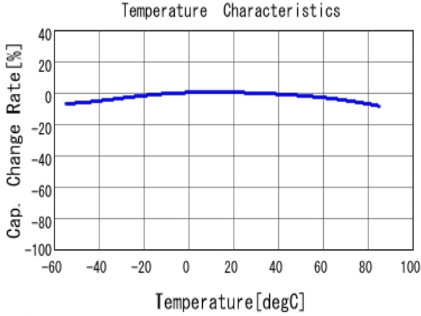
■ GRM033R61E104ME14 C-Temp. capchange, DCO. 0V, ACO. 5V rm
