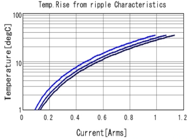
GRM033R61E104ME14 Temp. rise ■ 400kHz ■ 800kHz ■ 1MHz
