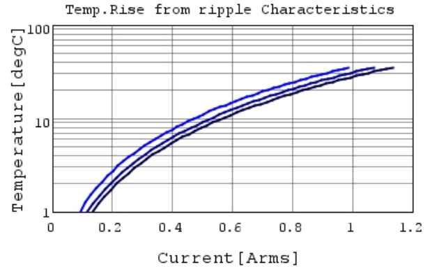
GRM033R61E104KE14 Temp.rise — 400kHz
