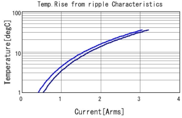
GRM033R61A225KE47 Temp. rise ■ 500kHz ■ 1MHz
