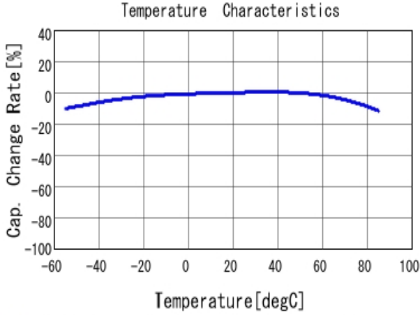
■ GRM033R61A224KE90 C-Temp. capchange, DCO. 0V, ACO. 2V rm
