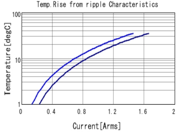
GRM033R61A224KE90 Temp. rise ■ 600kHz ■ 1MHz
