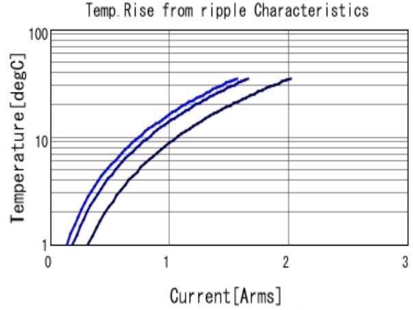
GRM033R60J474KE90 Temp. rise ■ 200kHz ■ 500kHz ■ 1MHz
