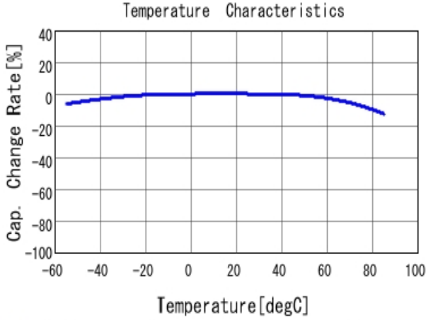
■ GRM033R60J474KE90 C-Temp. capchange, DCO. 0V, ACO. 2V rm
