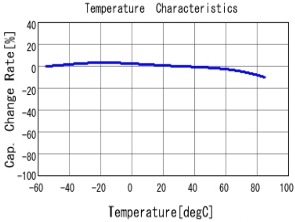
■ GRM033R60J224KE15 C-Temp. capchange, DCO. 0V, ACO. 5V rm
