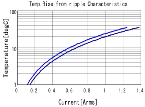
GRM033R60J224KE15 Temp. rise ■ 600kHz ■ 1MHz
