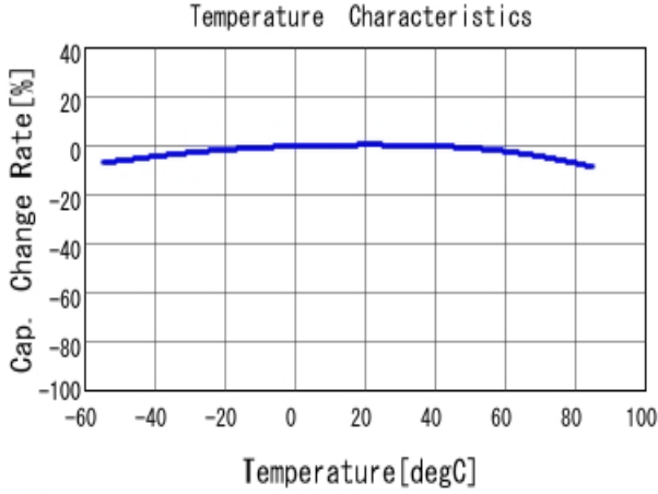
■ GRM033R60J153KE01 C-Temp. capchange, DCO. 0V, ACO. 5Vrm
