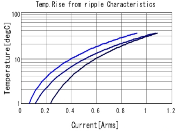
GRM033C71A104KE14 Temp. rise ■ 400kHz ■ 800kHz ■ 1MHz
