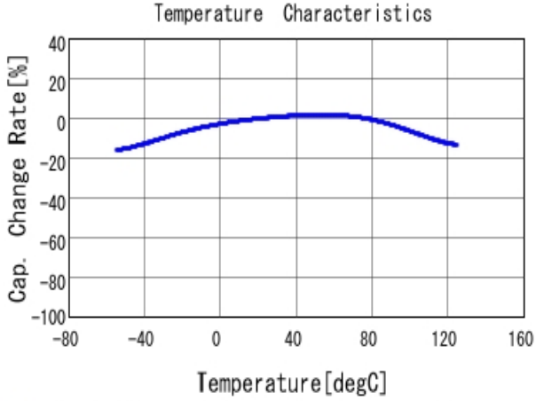
■ GRM033C71A104KE14 C-Temp. capchange, DCO. 0V, ACO. 2V rm
