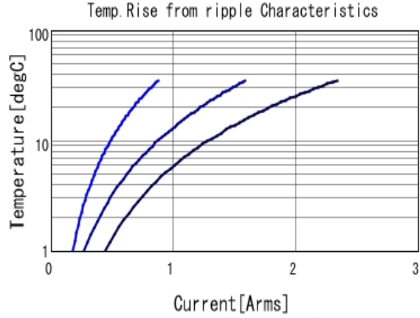
GRJ43DR72E474KWJ1 Temp. rise ■ 30kHz ■ 100kHz ■ 300kHz
