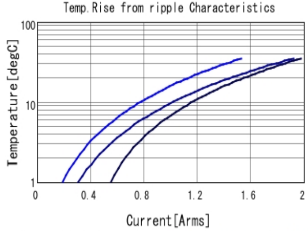
GRJ188R71H224KE11 Temp. rise ■ 300kHz ■ 600kHz ■ 1MHz
