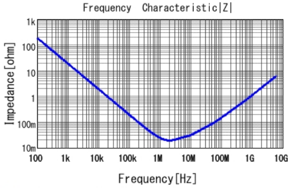
■ GRJ155R60J106ME11 |Z| DCOV, 25degC
