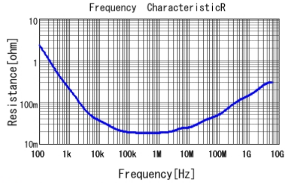
■ GRJ155R60J106ME11 R DCOV, 25degC
