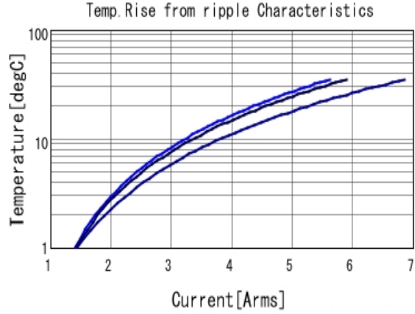
■ GCM32ER71E106KA57 Temp. rise ■ 80kHz ■ 400kHz ■ 800kHz
