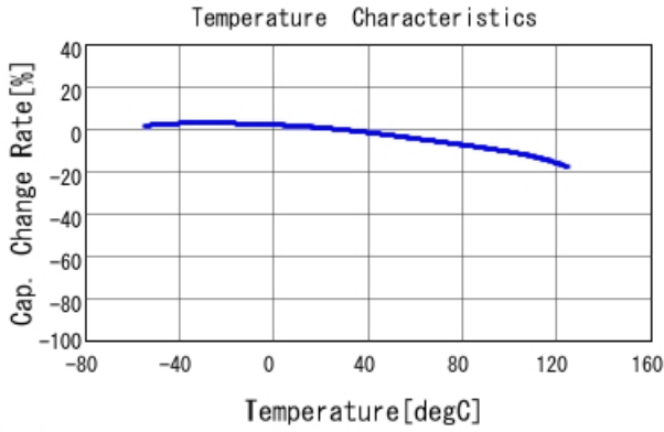
GCM32EC71H106KA03 C-Temp. capchange, DCO. 0V, AC1. 0Vrm
