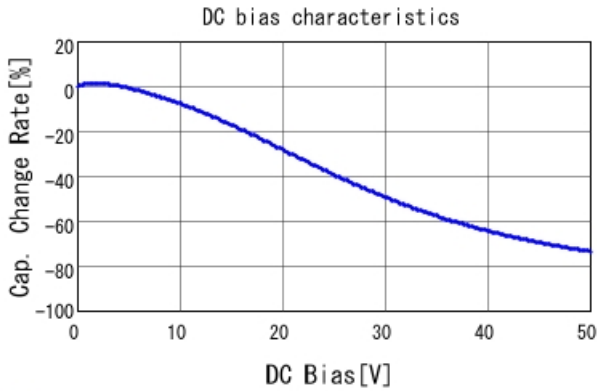
GCM32EC71H106KA03 C-DC bias capchange, 25.0degC, AC1.
