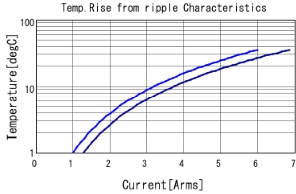
GCM32EC71H106KA03 Temp. rise ■ 80kHz ■ 400kHz
