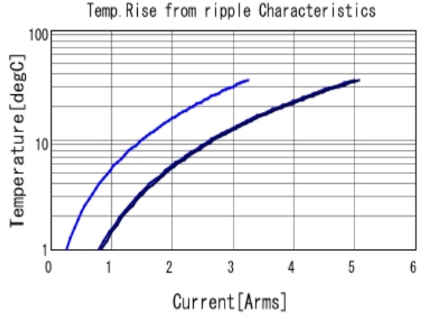
■ GCM31CR71C106KA64 Temp. rise ■ 80kHz ■ 400kHz ■ 800kHz
