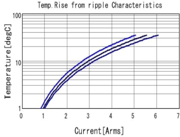
GCM31CC71E106KA03 Temp. rise ■ 80kHz ■ 400kHz ■ 800kHz
