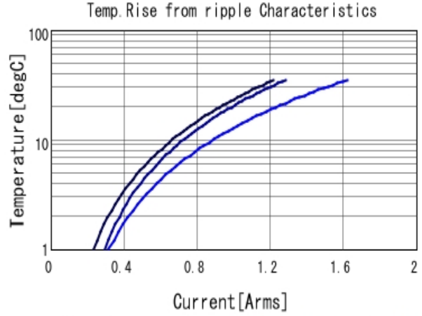
■ GCM21BR72A104KA37 Temp. rise ■ 400kHz ■ 800kHz ■ 1MHz
