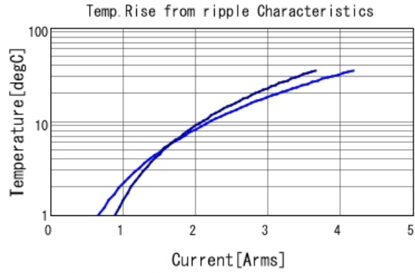
GCM21BR71H105KA03 Temp. rise — 500kHz — 1MHz
